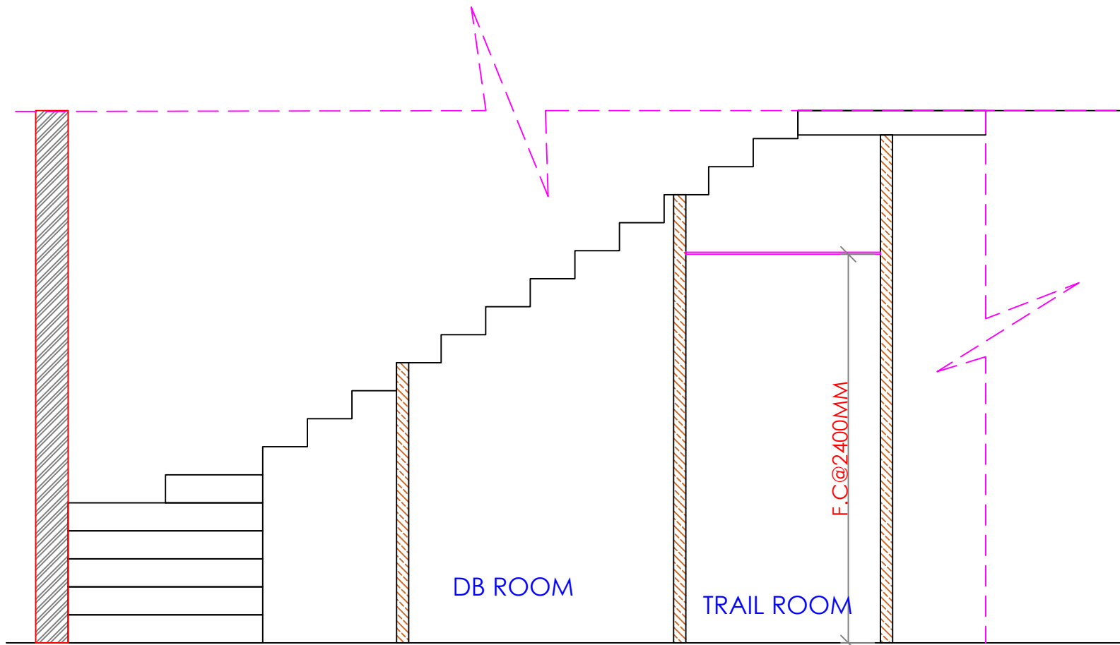
2 SECTION S2 Scale: NTS
