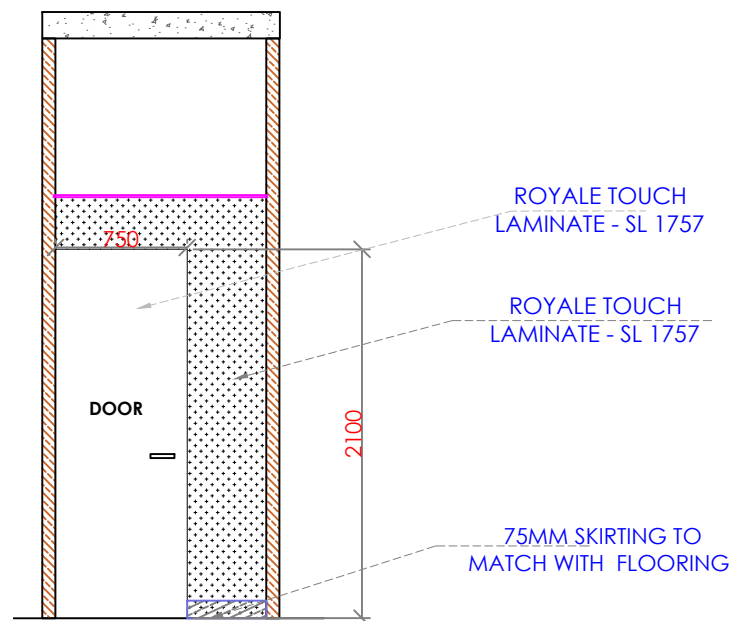
4 SECTION S4 Scale: NTS
