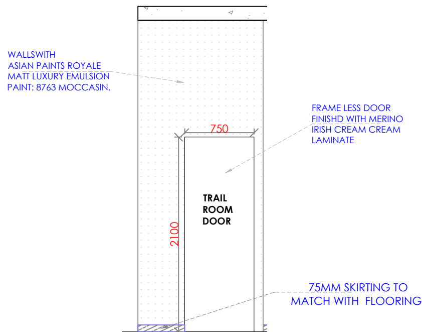
3 SECTION S3 Scale: NTS
